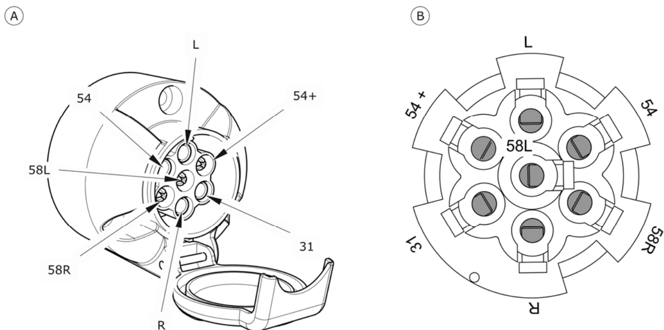
РИСУНОК 3.15 Разъем
